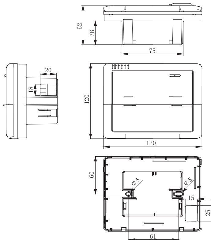
Рис. 6.20 Установочные размеры
